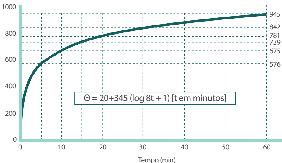
Figura 8 - Curva de crescimento da temperatura e forno de resistência ao fogo (Fonte: IPT).
