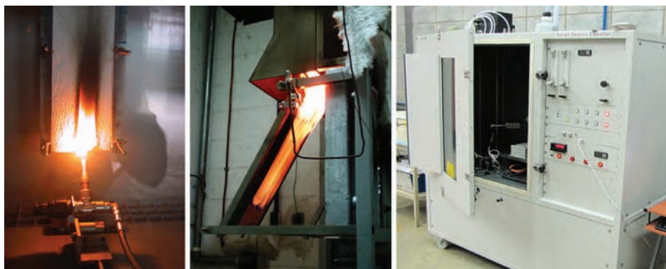
Figura 9 - Equipamentos para ensaios de ignitibilidade, propagação superficial de chamas e densidade óptica de fumaça (Fonte: IPT)
