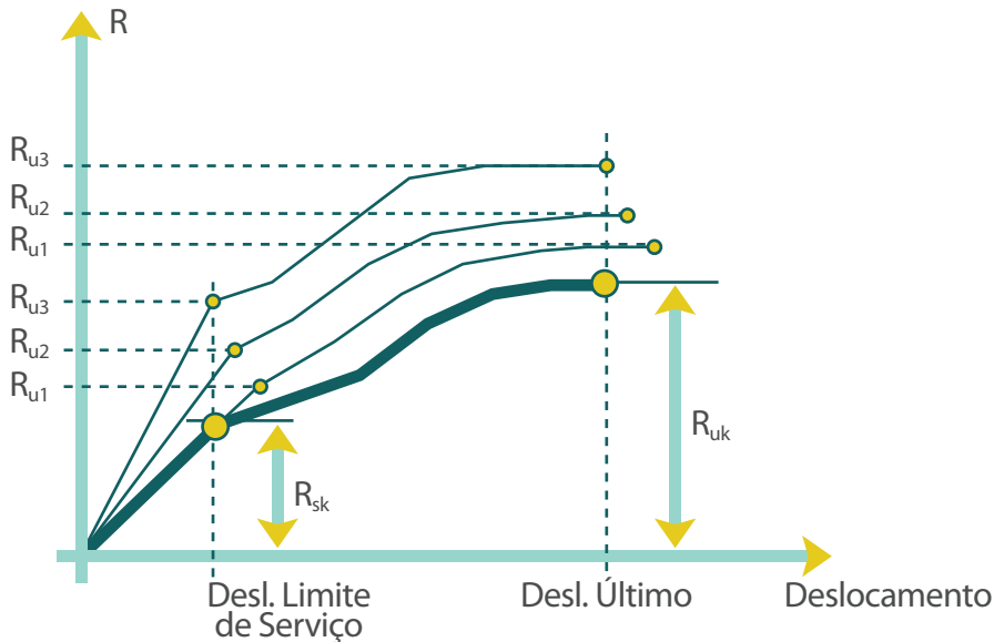
Figura 2 – Gráfico carga x deslocamento para determinação de R_{sd} e R_{uk} por meio de ensaios (Fonte: NBR 15.575-2)
