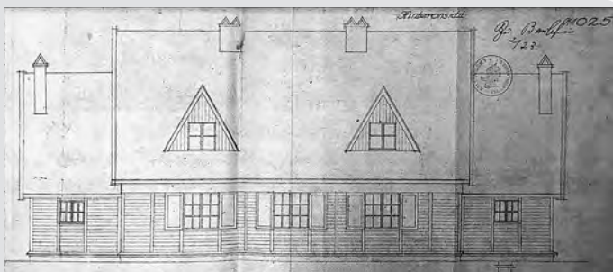
Hofansicht für das Zweifamilienhaus am Ziegelweg, Zeichnung zum Bauantrag, 21. Dezember 1922
